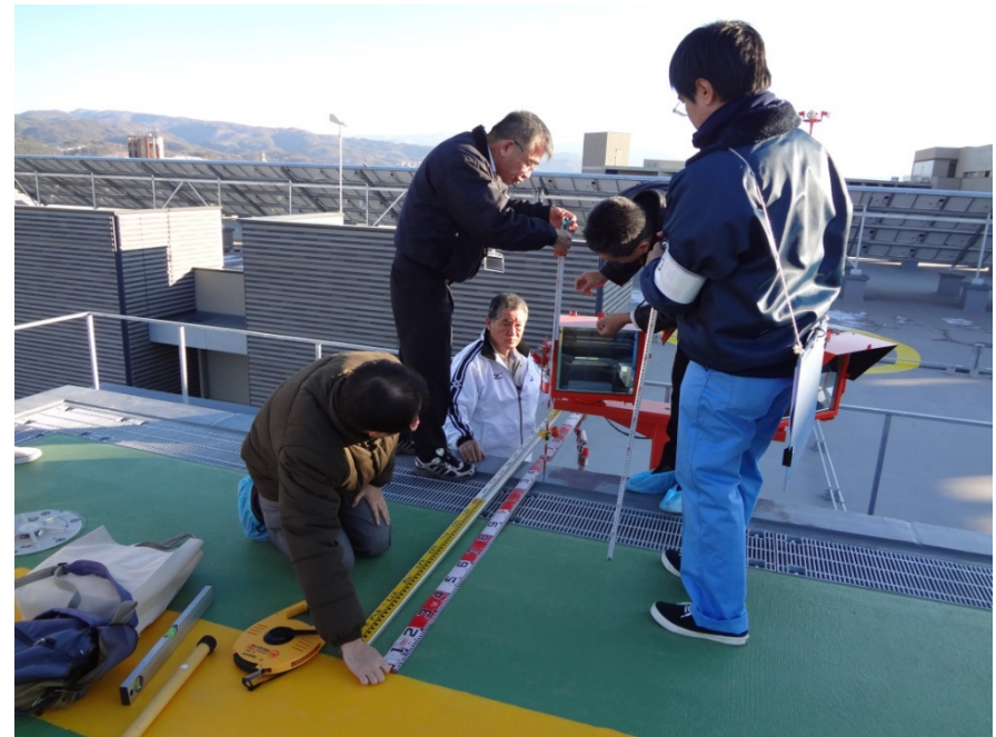
航空法に基づく制限値を満たしているか検査している様子 （佐久医療センターヘリポート（長野県））
