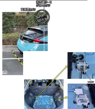
センサーの車両搭載状況(開発途中)
