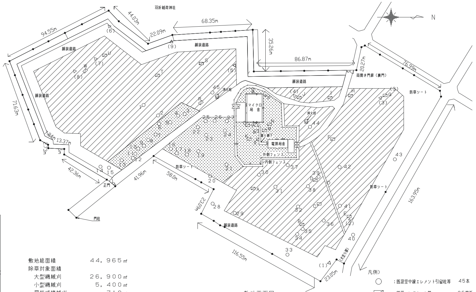
敷地平面図
