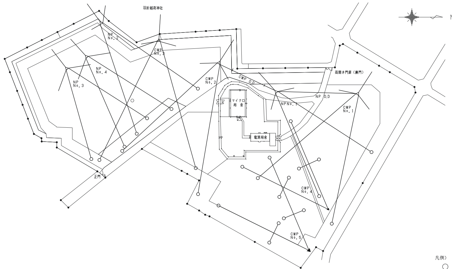
空中線配置図
