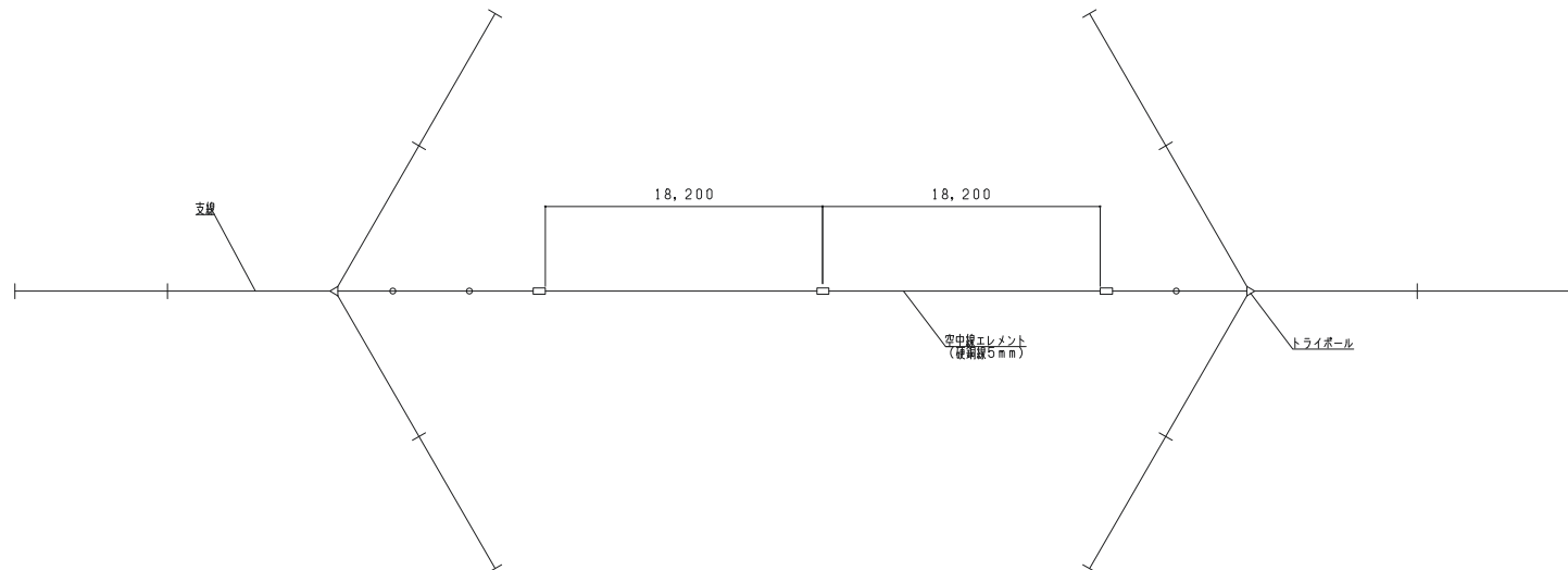
ダブル・ダブルレット空中線（CWP）展張図
