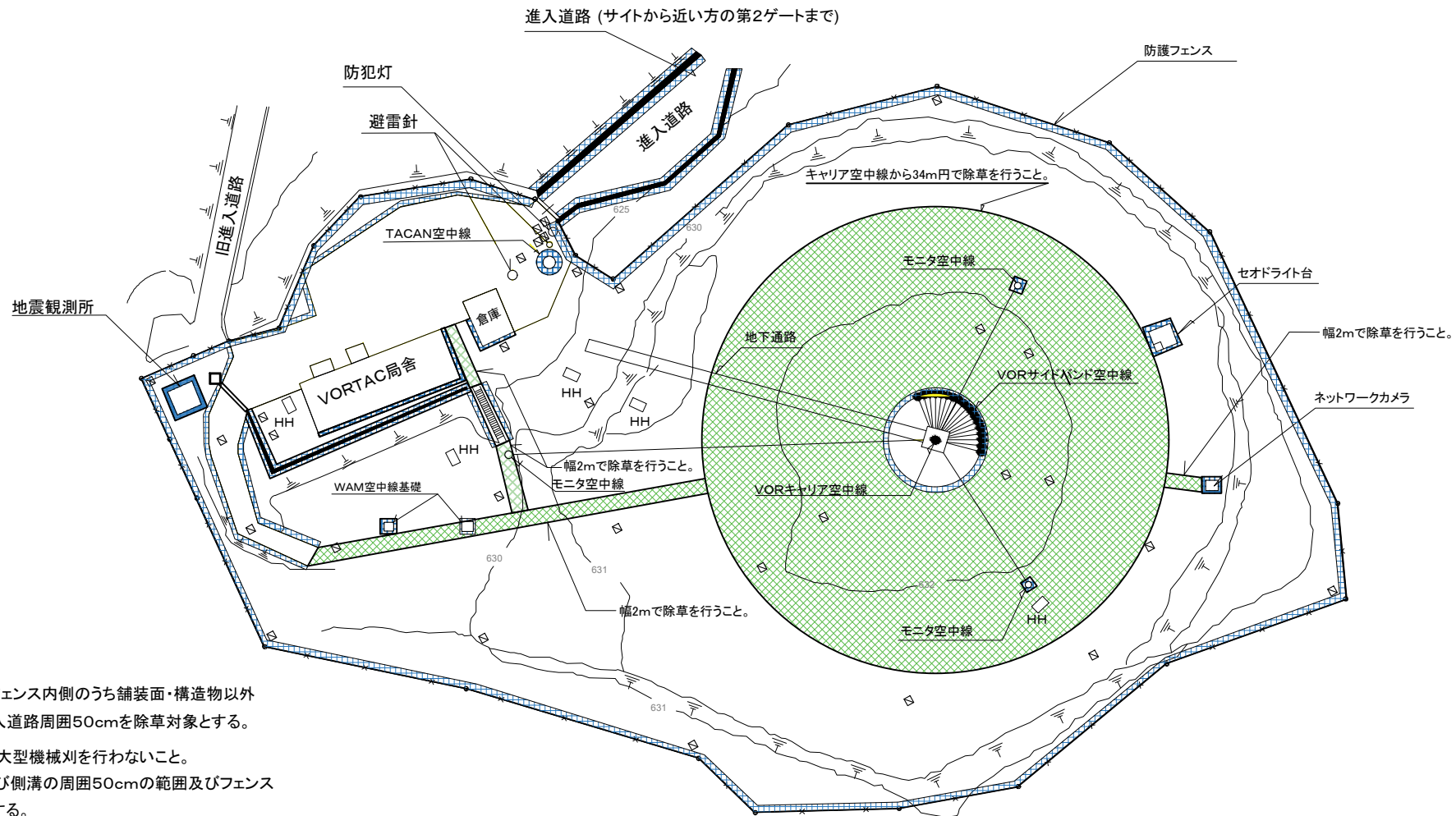
大島VORTAC 敷地平面図
