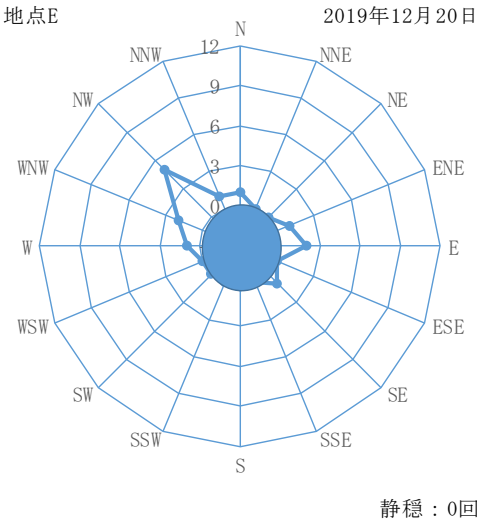
図 4-4 (8) 風配図 (8)
