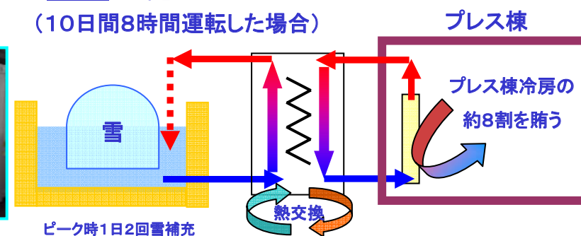
移動式雪冷熱冷房装置
