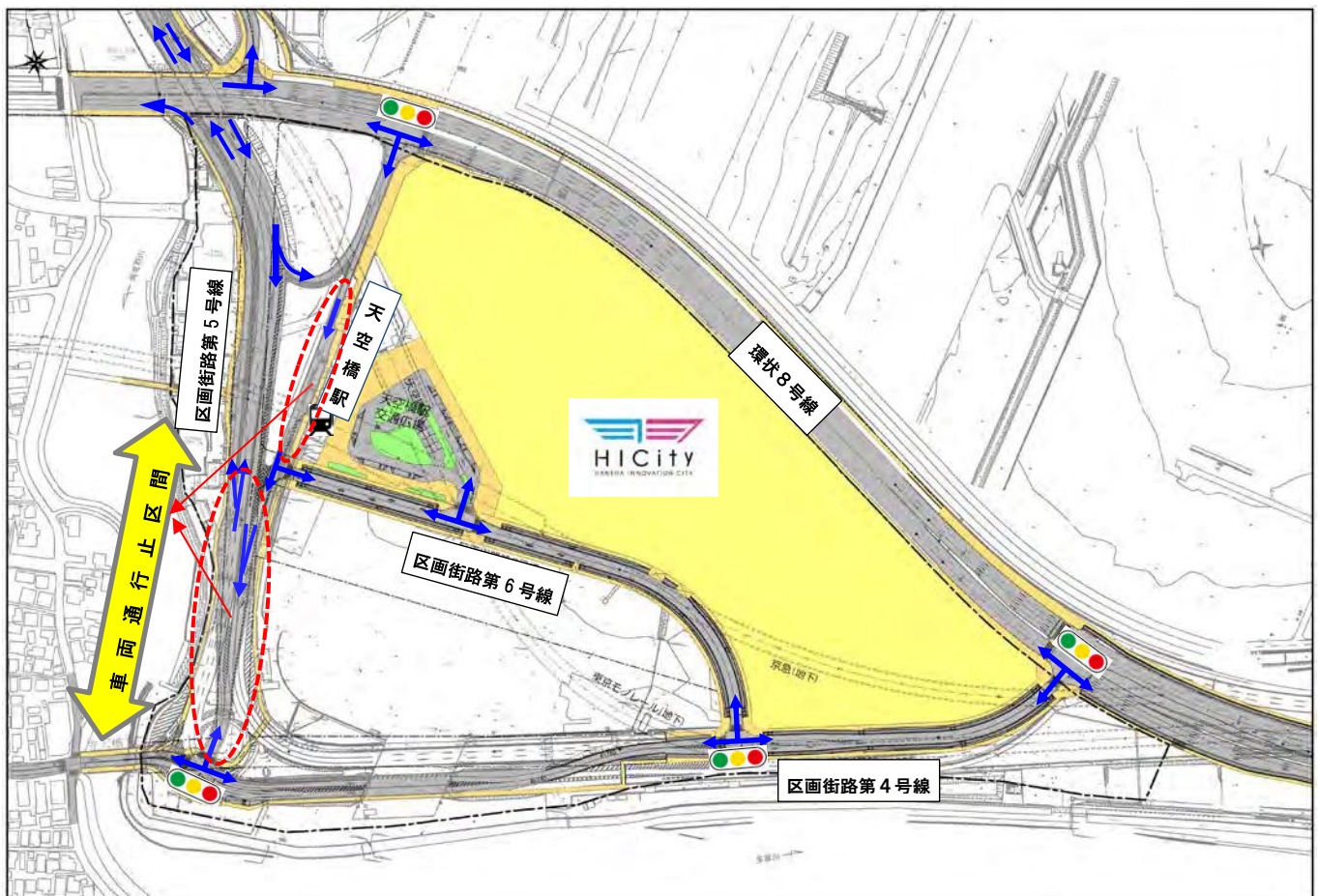
現況道路平面図
