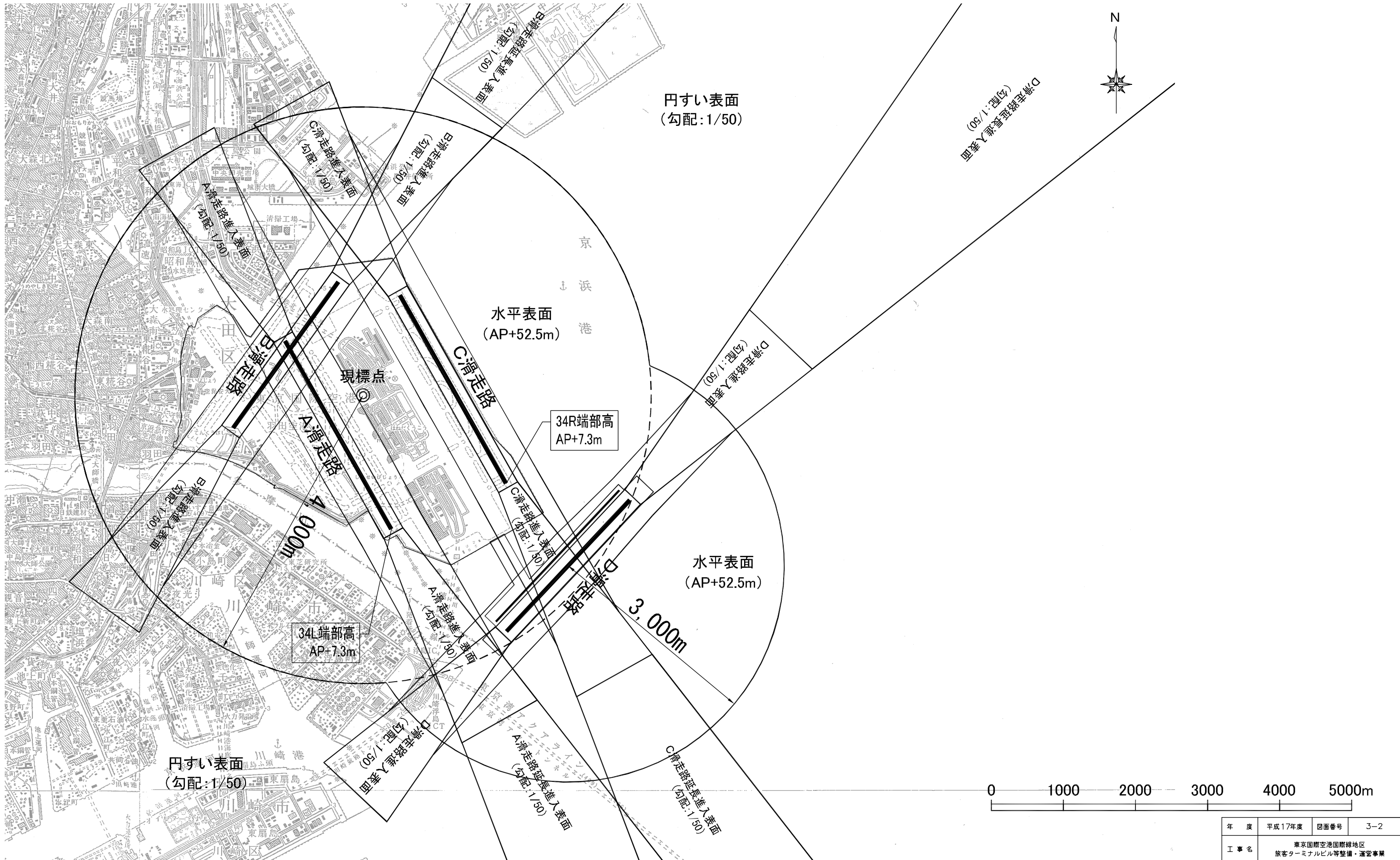
再拡張後の予定制限表面図
