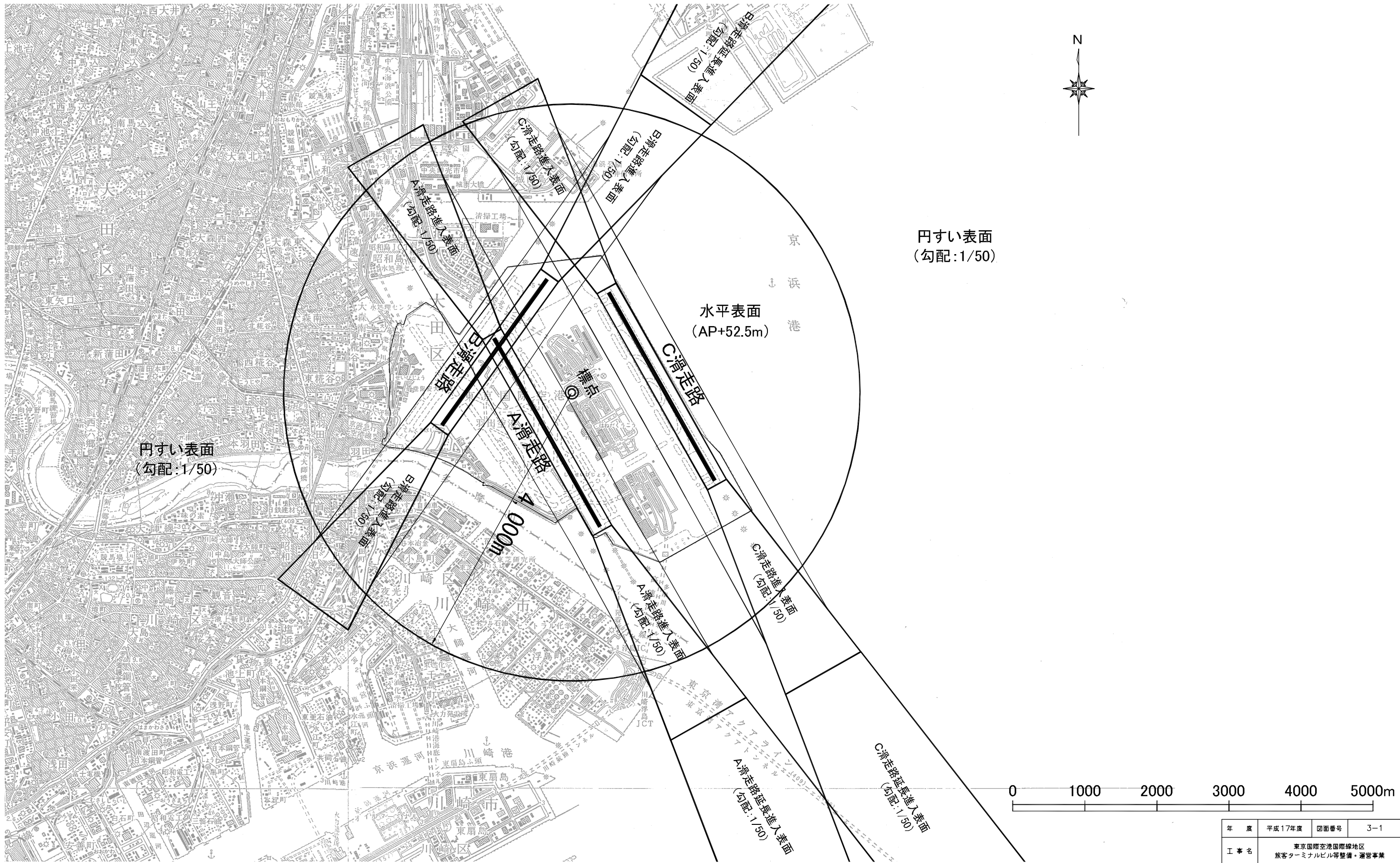
現況の制限表面図
