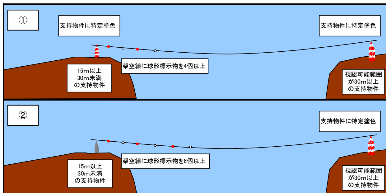
図5-15 両端の支持物件の水平間隔が700m以下の場合の具体例（その1）
