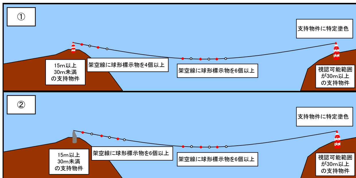
図5-17 両端の支持物件の水平間隔が700mを越える場合の具体例（その1）
