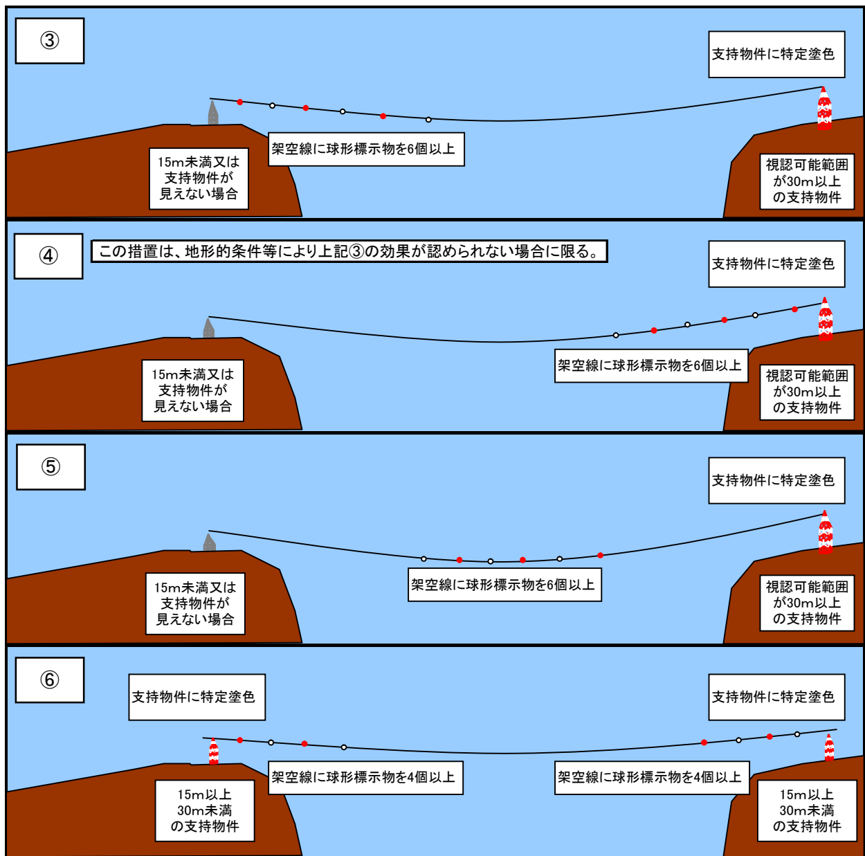
図5－16 両端の支持物件の水平間隔が700m以下の場合の具体例（その2）
