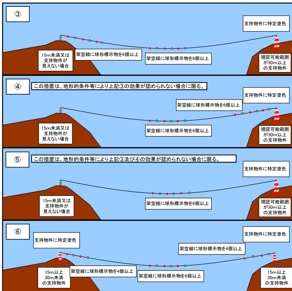
図5-18 両端の支持物件の水平間隔が700mを越える場合の具体例（その2）
