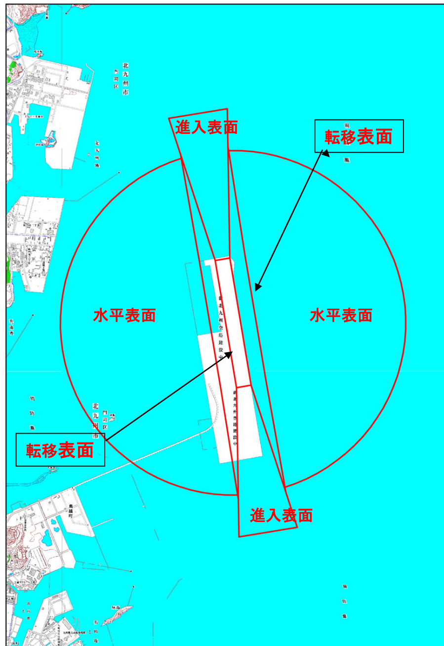
新北九州空港の制限表面区域図
